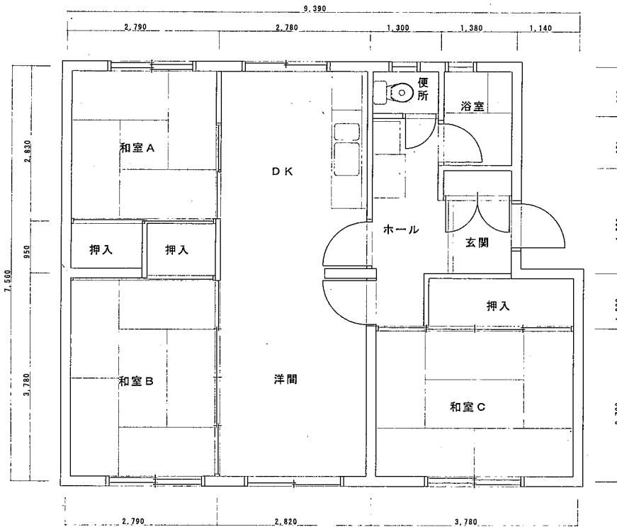
職員宿舎7号棟各戸平面図 S=1:100
